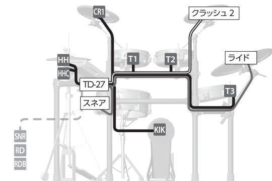
図 B：TD-27KV 背面から見た図
