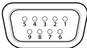
9ピン D-sub タイプ (メス)
