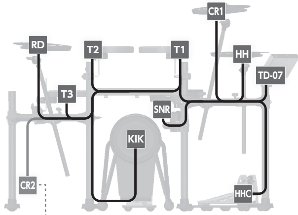
専用接続ケーブル配線図 （背面から見た図）
